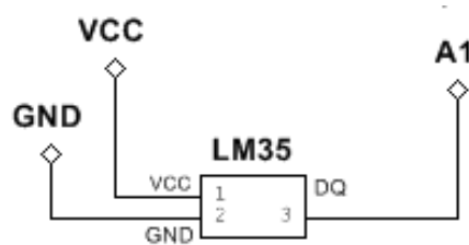
Figura 13: Circuito medición de Temperatura
