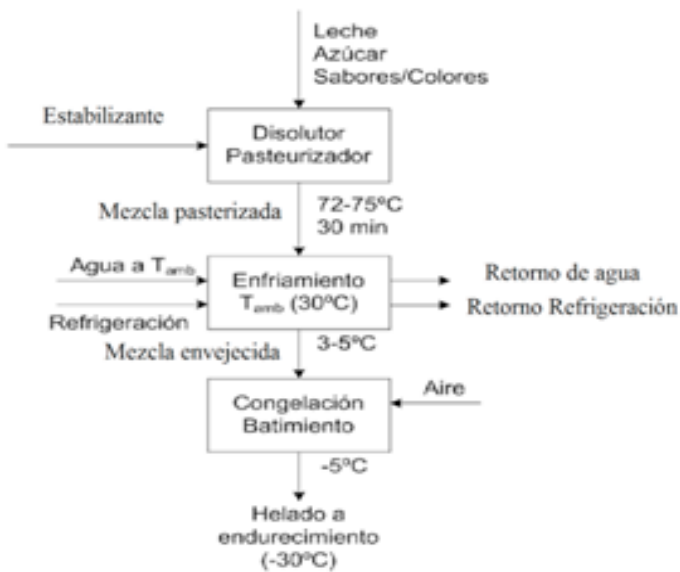
Figura 2: Esquema del proceso empleado para la producción de helados a escala piloto.
