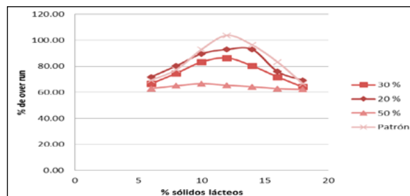
Figura 6: Comportamiento del rendimiento con la sustitución de estabilizador Brigel Neutro Trial por almidón modificado para diferentes contenidos de sólidos.
