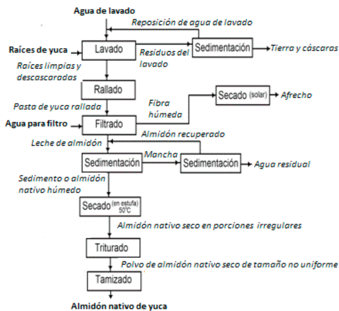
Figura1: Procedimiento seguido para la obtención del material de partida.
