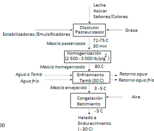
Figura 3. Esquema del proceso utilizado en la prueba industrial.
