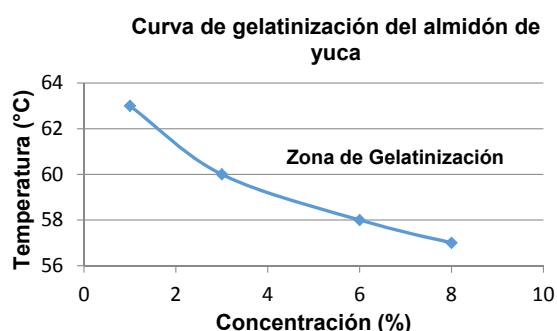
Figura 4: Curva de gelatinización de suspensiones de almidón nativo de yuca.
