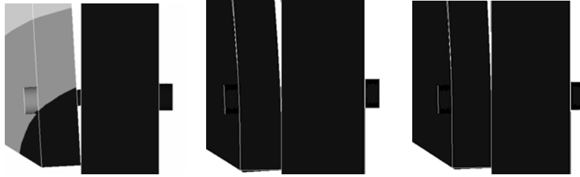
Şekil 4 En alttaki civatanın deformasyonu (100 defa büyütülmüş halleri) a) Rijit elemanlar b) Elastik elemanlar c) Elastik elemanlar ve 0.04 mm sıkılmış civatalar.
