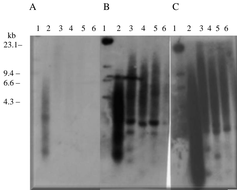
Fig. 10. Comparative Southern hybridization of S. bicolor (SBI-02) BACs (A) 112a4, (B) 48d12 and (C) 109b1 to genomic DNA of S. bicolor (lane 2), S. angustum (lane 3), S. versicolor (lane 4), S. brachypodum (lane 5) and S. intrans (lane 6). \lambda - Hind III marker (lane 1) serves a molecular marker and control.
