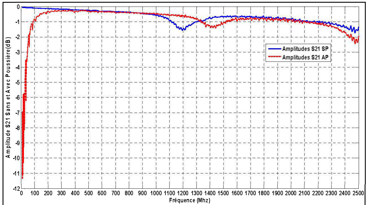
Figure 4.22: Mesures du paramètre S_{21} au laboratoire
