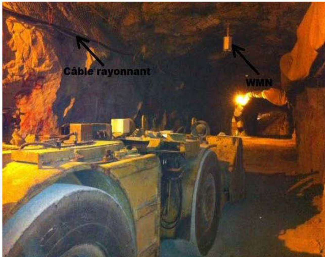
Figure 2.4: Exemple des infrastructures installées dans une mine souterraine
