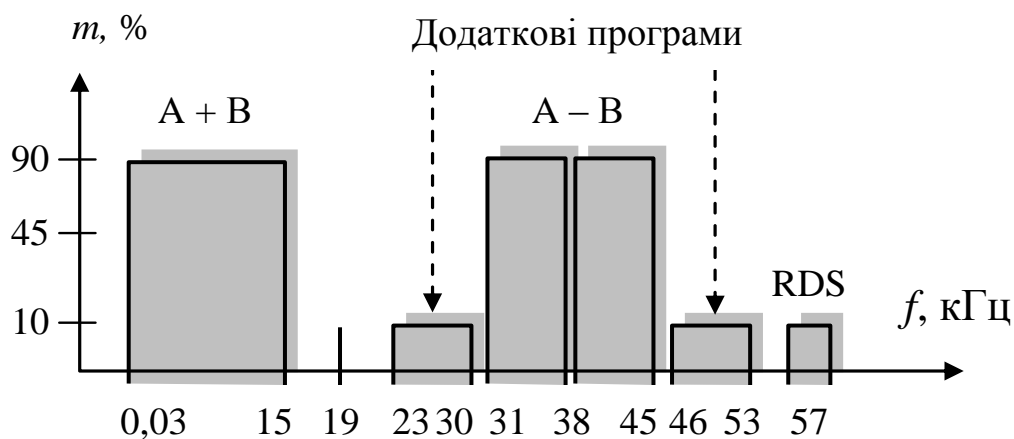
Рис. 1. Спектр складеного стереофонічного сигналу за способом аналого-цифрового мовлення у діапазоні ДВЧ
