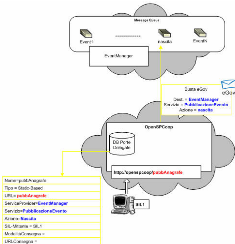
Figura 2-12, Scenario di utilizzo di una porta delegata registrata per la pubblicazione di un evento
