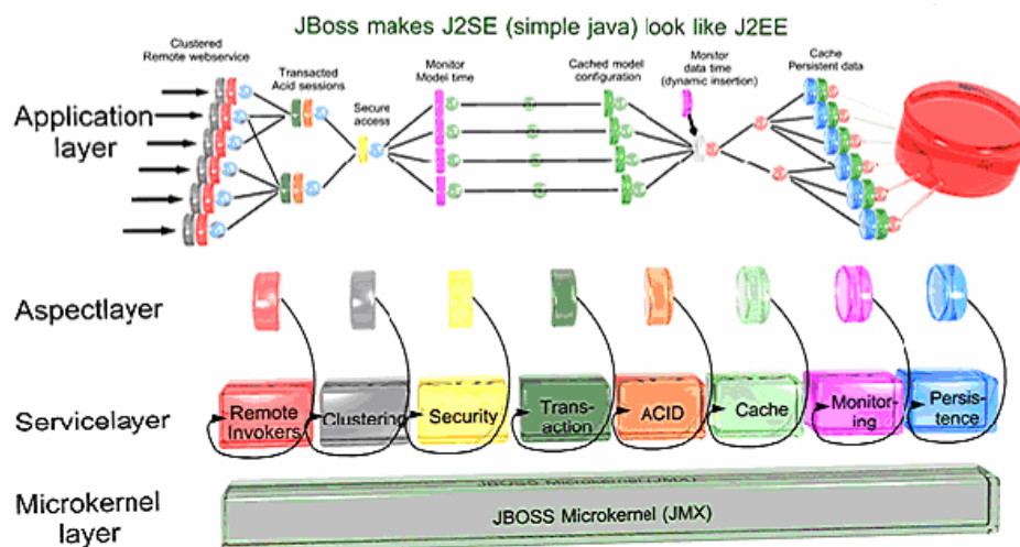
Figura 3-2, Architettura dell'application server JBoss
