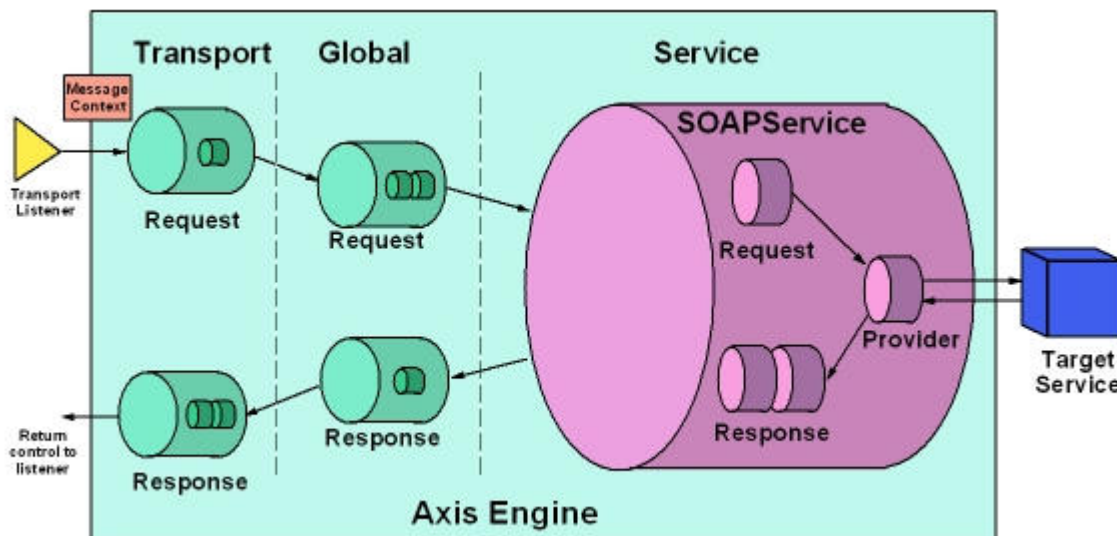
Figura 3-5, Architettura a pipeline del prodotto Apache Axis
