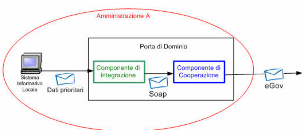
Figura 1-14, Visione 'classica' del CNIPA per la Porta di Dominio (Componente di Integrazione e Componente di Cooperazione)
