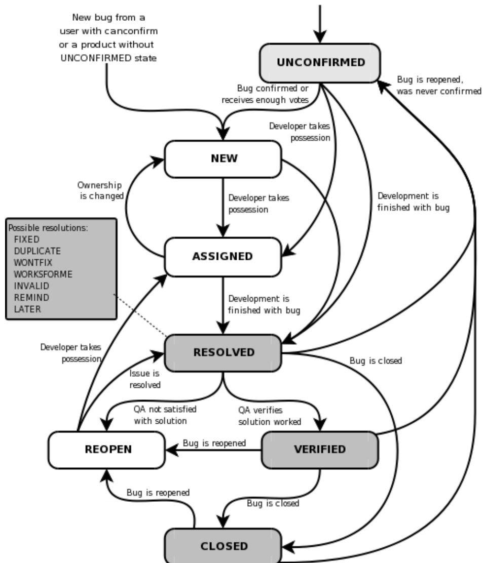
Figura 4-2, Il Ciclo di Vita di un Bug per Bugzilla
