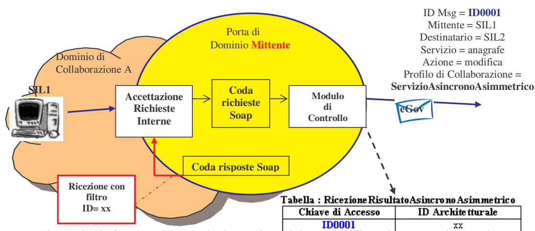
Figura 2-43, Gestione di una richiesta di servizio con profilo asincrono asimmetrico
