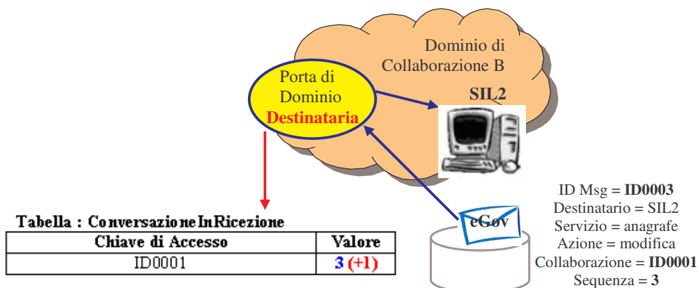
Figura 2-31, Scongelo di buste precedentemente congelate poiché arrivate fuori ordine.
