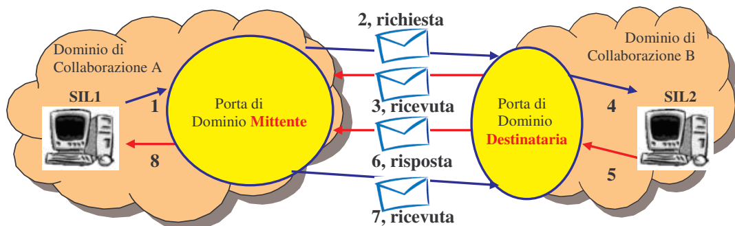
Figura 2-37, Flusso delle buste SPCoop scambiate durante un profilo asincrono simmetrico
