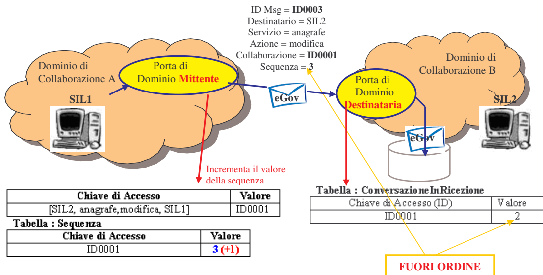
Figura 2-29, Scenario in cui una porta di dominio riceve una busta, appartenente ad una conversazione, non in ordine.
