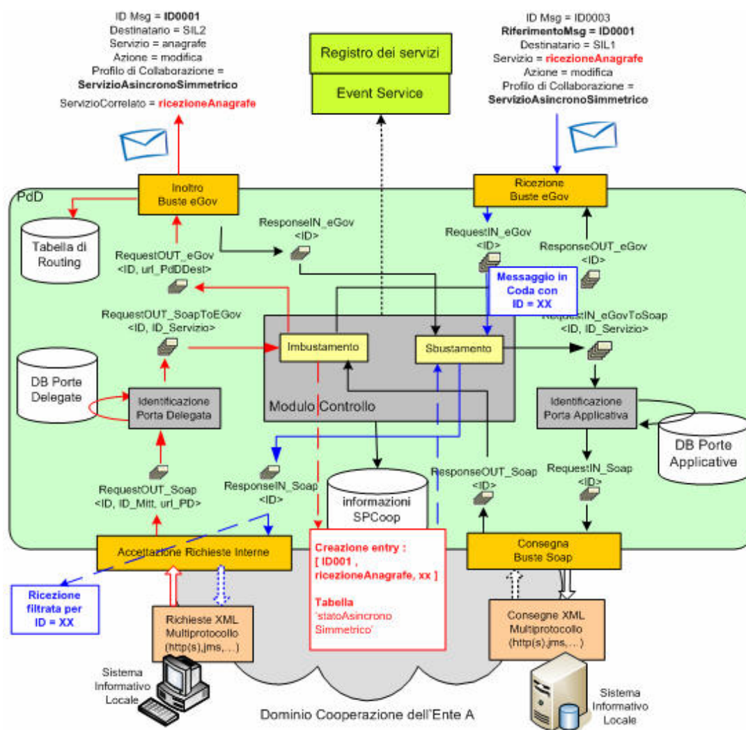
Figura 2-38, Gestione del profilo asincrono simmetrico all'interno dell'architettura di una porta di dominio che riveste il ruolo 'mittente'
