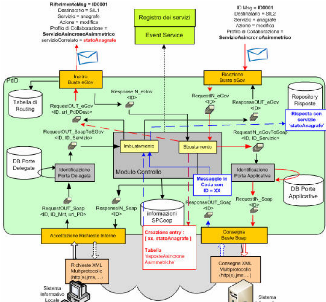
Figura 2-47, Gestione del profilo asincrono asimmetrico all'interno dell'architettura di una porta di dominio che riveste il ruolo 'destinatario'
