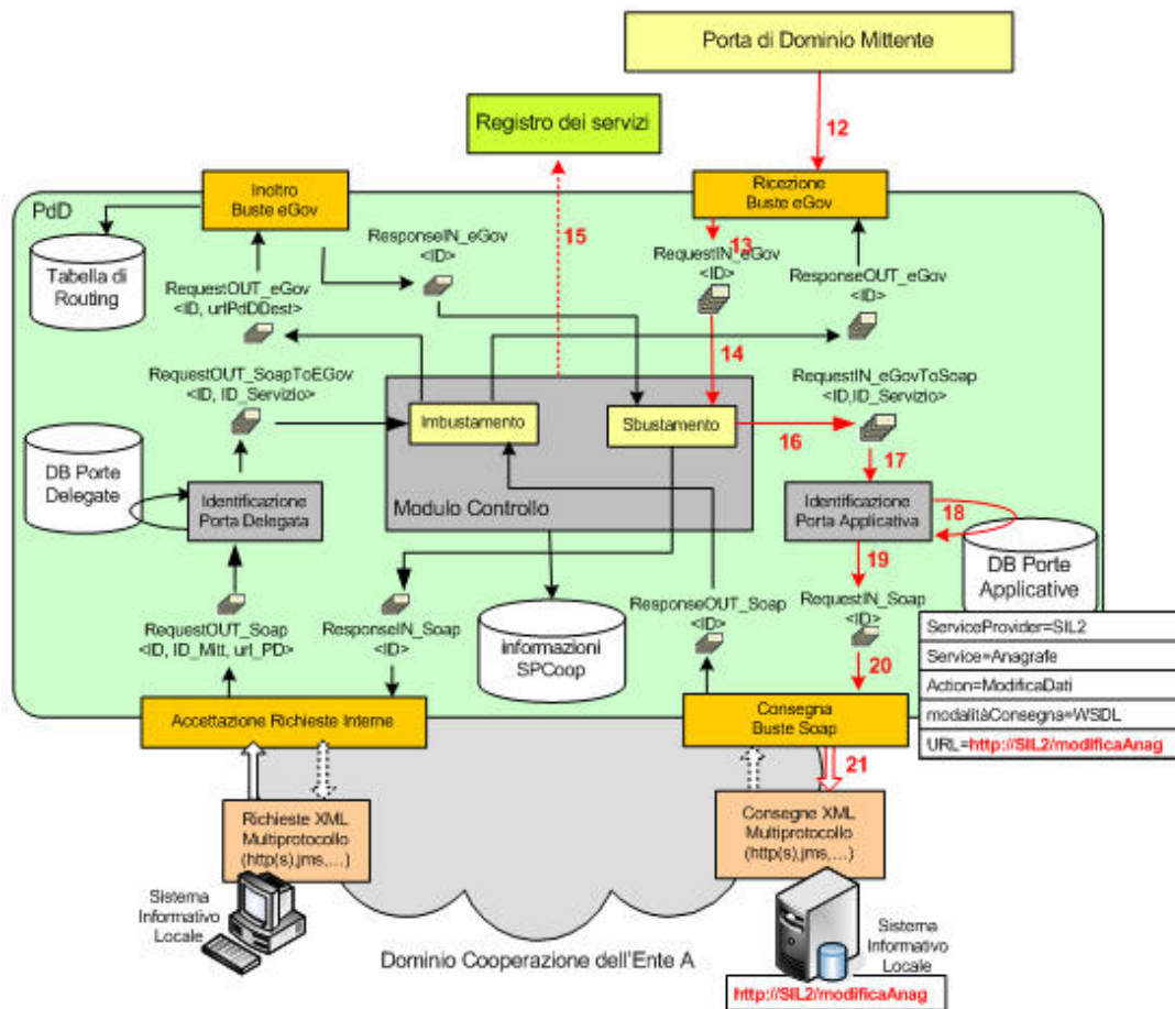
Figura 2-55, Gestione dell'invocazione di Servizio effettuata all'interno dell'architettura di una porta di dominio 'Destinataria'
