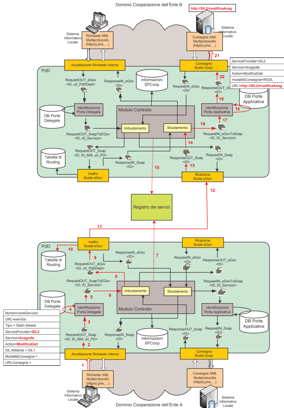
Figura 2-56, Caso d'uso completo di invocazione di un servizio
