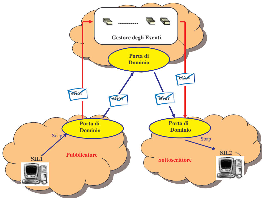
Figura 2-11, Scenario di una cooperazione applicativa ad eventi in OpenSPCoop
