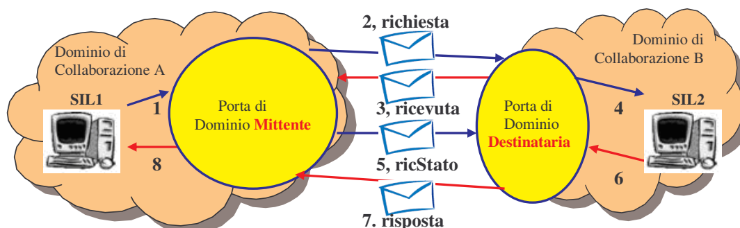
Figura 2-42, Flusso delle buste SPCoop scambiate durante un profilo asincrono asimmetrico
