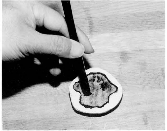
図91 乾漆による欠損刳足部分の製作 Making the missing part of the kuriashi with kanshitsu
