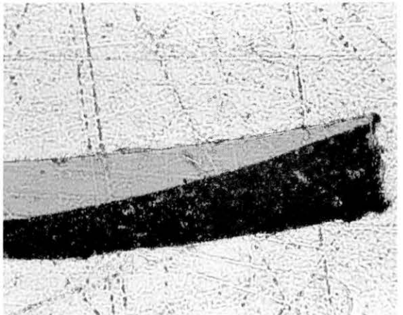
図107 中塗・上塗漆のクロスセクション Cross section of the middle coating and final coating
