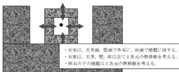
図2 計算対象
