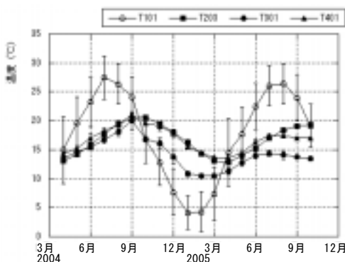
図4 発掘開始後の月平均温度変化 T101：外気 T203：地温 T301：小前室 T401：石室内
