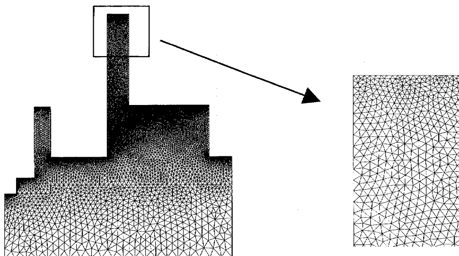
図8 レンガ構造物のメッシュ図
