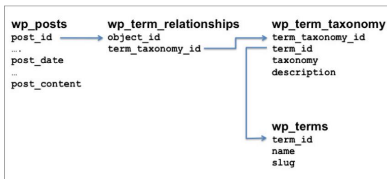
Рис. 1. Связи таблиц базы данных CMS Wordpress, содержащих данные о записях и терминах таксономии
