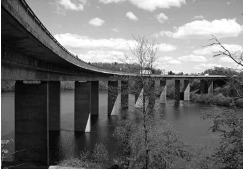
Abb. 1: Die Brücke über dem Biggesee. – The motorway bridge above the Biggesee.
