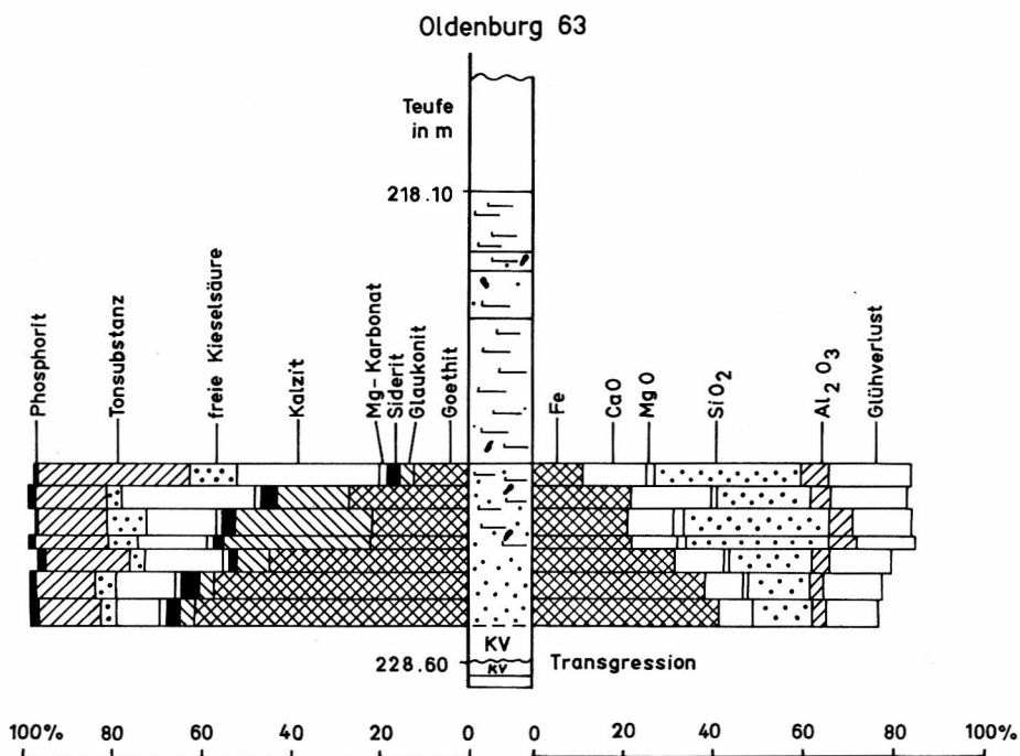
Abb. 10 Mineralbestand und Chemismus des Campan-Eisenerzes in der Bohrung Oldenburg 63 (Karte 1:25000, Bl. 3414 Holdorf, R 3442910, H 5823829; vgl. Abb. 6 und 8). Nach JANSEN (1962)
