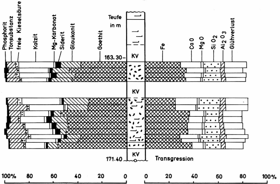
Abb. 9 Mineralbestand und Chemismus des Campan-Eisenerzes in der Bohrung Oldenburg 60 (Karte 1:25000, Bl. 3414 Holdorf, R 3442958, H 5824413; vgl. Abb. 4, 6 und 8). Nach JANSEN (1962)
