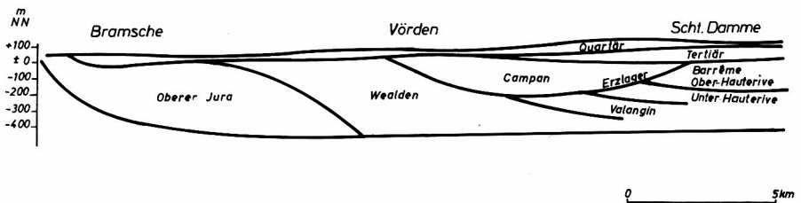
Abb. 3 Geologische Übersichtskarte und SW-NE-Schnitt der „Dammer Oberkreide-Mulde“ mit den Eisenerzvorkommen Damme, Gehrde und Rieste (nach Unterlagen der früheren Erzbergbau Porta-Damme GmbH entworfen von ROLF THIENHAUS). Stemmer Berge = Stemmweder Berge
