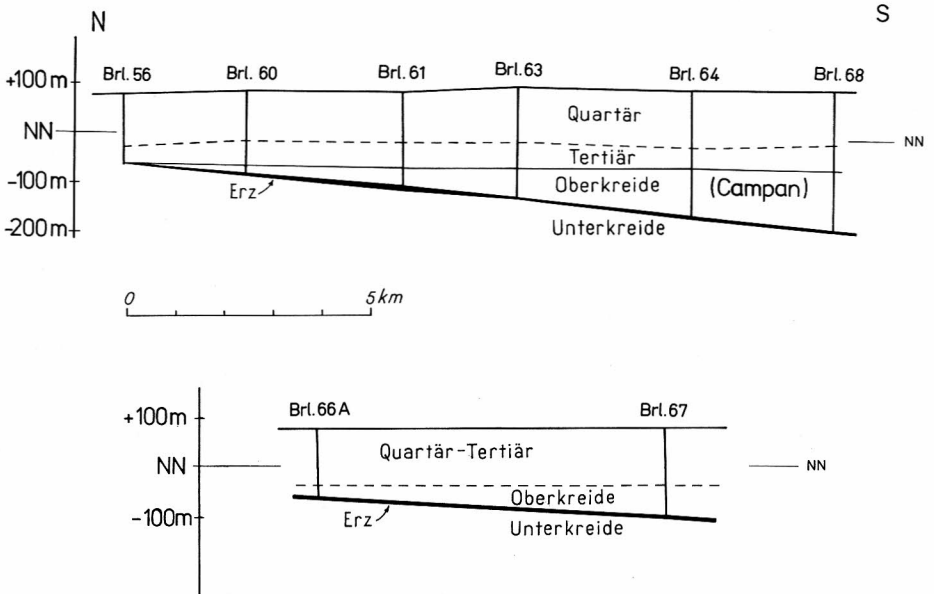
Abb. 6 N-S-Schnitte (Querprofile) durch den Nordflügel der „Dammer Oberkreide-Mulde“. Lage der Bohrungen (vgl. Abb. 4): Karte 1 : 25 000, Bl. 3414 Holdorf: Oldenburg 56, R 34 42 871, H 58 24 717; Oldenburg 60, R 34 42 958, H 58 24 413; Oldenburg 61, R 34 42 800, H 58 24 133; Oldenburg 63, R 34 42 910, H 58 23 829; Oldenburg 64, R 34 42 629, H 58 23 558; Oldenburg 68, R 34 42 667, H 58 23 227; Karte 1 : 25 000, Bl. 3415 Damme: Oldenburg 66 A, R 34 47 666, H 58 22 624; Oldenburg 67, R 34 47 388, H 58 21 962
