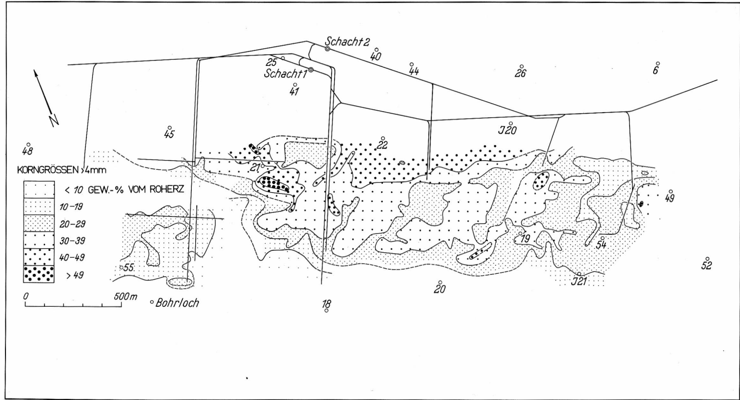
Abb. 12 Anteil der Körner über 4 mm Größe (in Gew.-% des Roherzes) im Campan-Eisenerz der Dammer Westlinse in der Umgebung der ehemaligen Doppelschachanlage Damme. Nach NEUMANN (1961)
