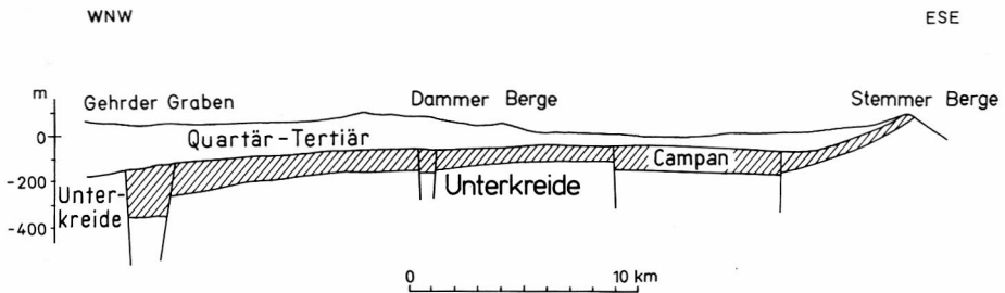
Abb. 7 Schematischer WNW-ESE-Schnitt (Längsprofil) durch den Nordflügel der „Dammer Oberkreide-Mulde“ von Gehrde bis zu den Stemmer Bergen (= Stemweder Bergen; vgl. Abb. 3, 4 und 5)
