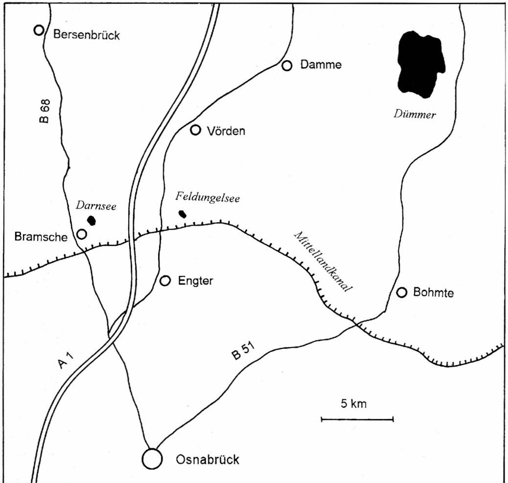
Abb. 1: Lage des Feldungelsees östlich der Straße Engter – Vörden, nördlich des Mittellandkanals. Fig. 1: Location of the Feldungelsee east of the road Engter – Vörden, north of the Mittellandkanal.
