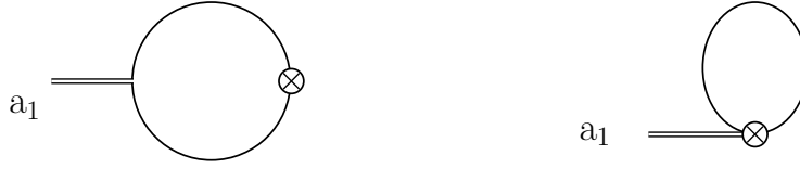
Figura 4.1: Representación diagramática de las contribuciones a la constante de decaimiento débil del pion provenientes del campo vectorial-axial.
