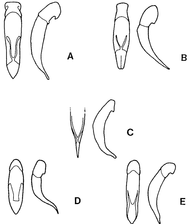
Figure 4. Microscelida spp., dorsal and lateral views of aedeagi. a) M. foveicollis , new species; b) M. subglabrata (Jacoby); c) M. whitingi , new species; d) M. moweryi , new species; e) M. violacea (Jacoby).
