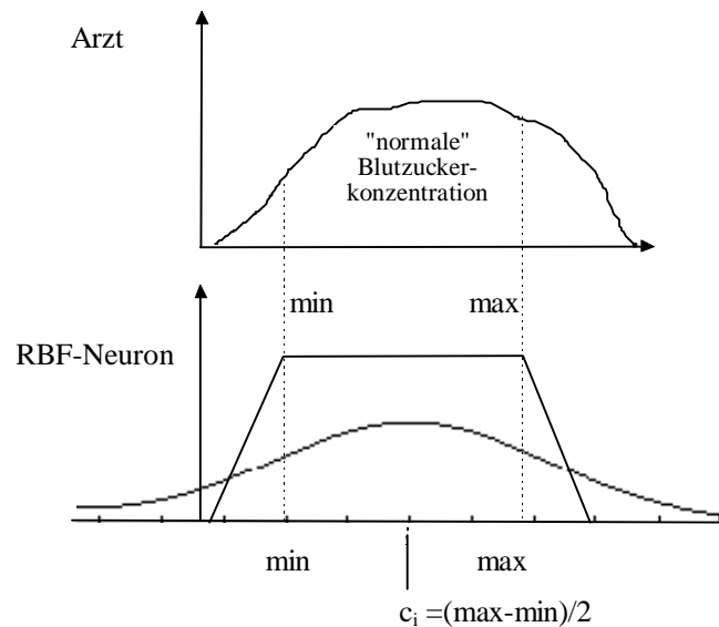
Abbildung 8 Initialisierung der RBF-Parameter mit dem Arztwissen
