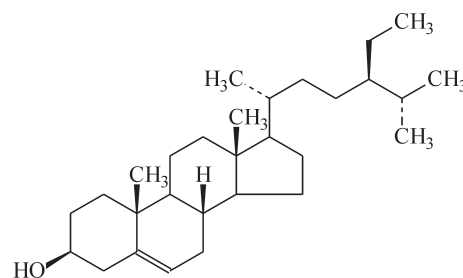
Fig. 1. \beta -Sitosterol (BSS).
