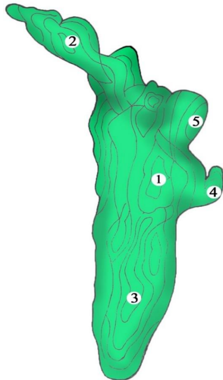
Рис. 2. Реконструкція сечово-статевої пазухи передплода 20,0 мм ТКД. Вигляд зліва. Графіка. Зб. 60: 1 – сечово-статева пазуха; 2 – сечовий міхур; 3 – сечівник; 4 – мезонефральна протока; 5 – сечовід
