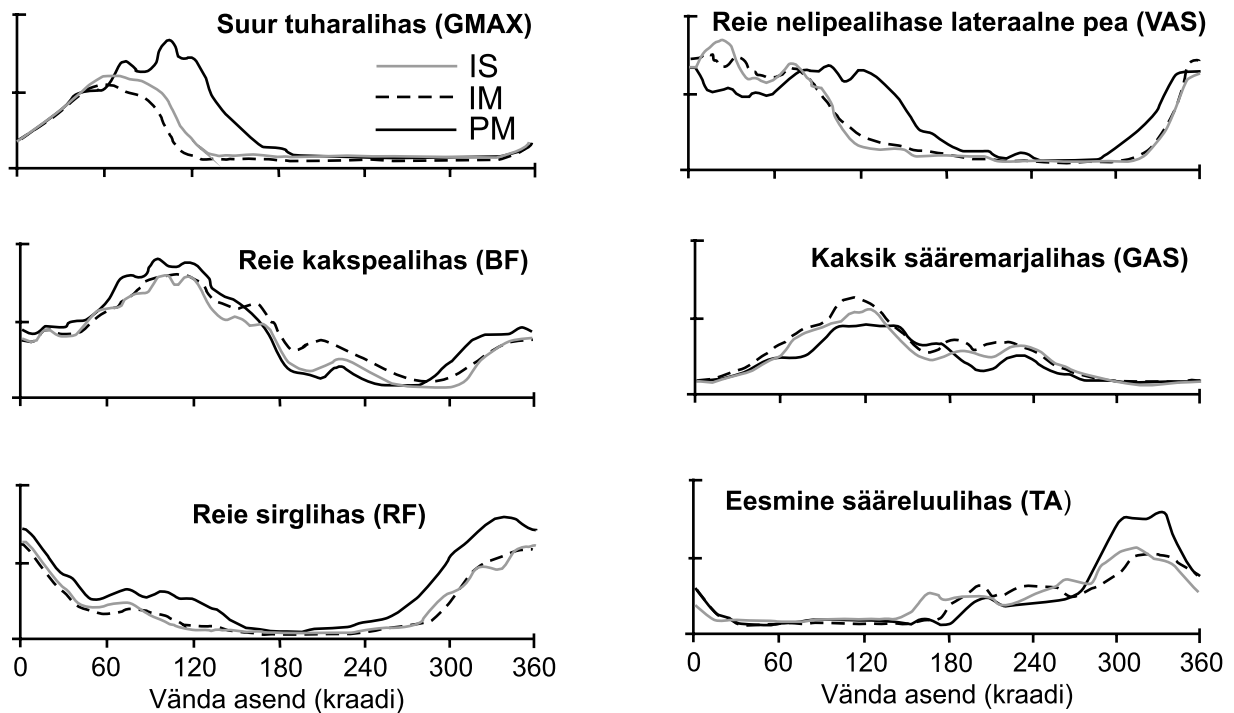
Joonis 44. Kuue olulisema lihase integreeritud EMG istes siledal-õidu asendis (IS), istes mækkesõidu asendis (MI) ja mække püstisõidu asendis (MP) kogu pedalleerimistsükli vältel, alustades ülemisest surnud punktist (Li ja Caldwell'i 1998).
