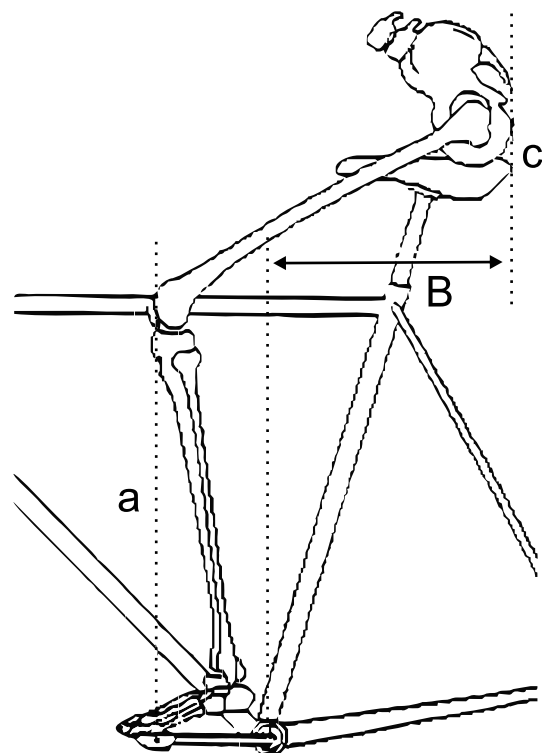
Joonis 6. Sadula tagaosa (c) horisontaalkaugus jalgratta keskjooksust (B), sõltuvalt põlve vertikaalsest asendist (a) pedaalil võlli tsentri suhtes vända asendis 90°.
