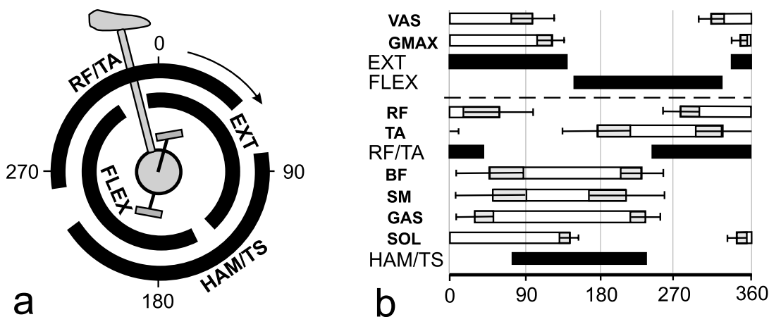
Joonis 43. Pedalleerimisel osalevate lihaskomplektide antagonistlikud paarid (A) ja "lihaskomplektide" jõurakendusmomendid (B) (Raasch et al. 1999 andmetel).
