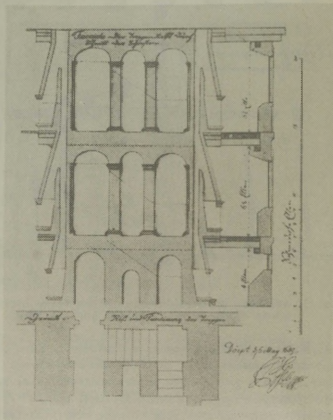
Joon. 6. Academia Gustavo-Carolina hoone trepikoja läbilõige 1690. a. P. v. Esseni joonise järgi.
