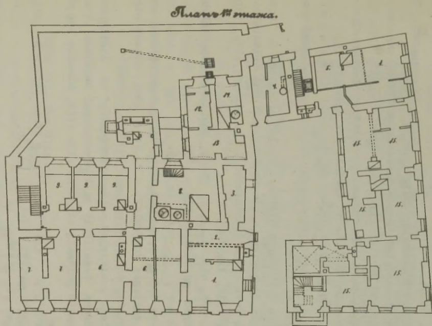
Joon. 9. Kruntidel numbriga 60 ja 61 asunud ehitised. Arhitekt R. Guleke 1886. a. (RAKA, f. 298, nim. 3, s.-ü. 484, l. 4.)
