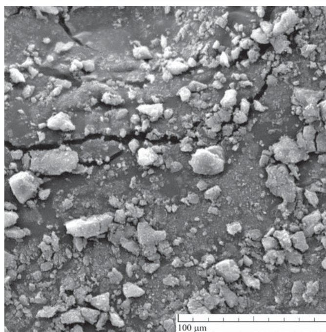
SLIKA 7 – Mikrografija površine čađe nakon obrade s \text{HNO}_3
