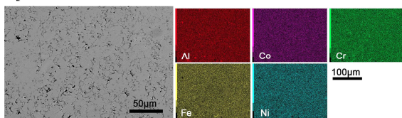
g Al 2 CoCrFeNi sintered powder - 2.1 GPa, 1253 K, 1h
