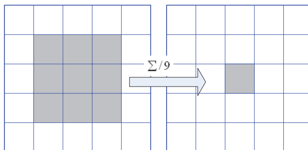
Slika 3. Filtar usrednjavanja
