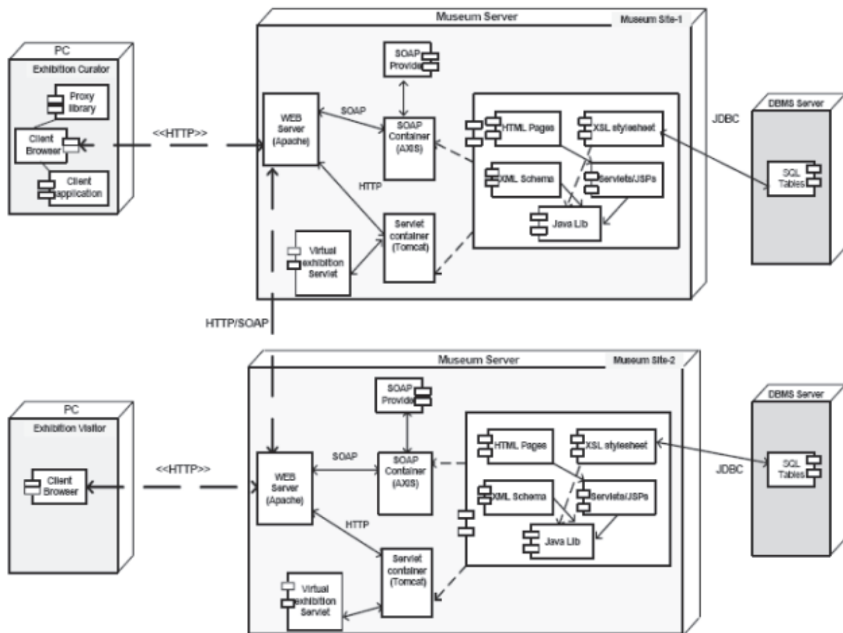
Slika 7. Razvojni dijagram
