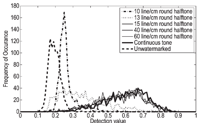
Figure 10 Histogram of detection values for a round halftone Slika 10. Histogram detektiranih vrijednosti za točkasti raster
