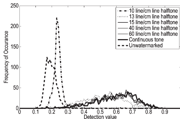
Figure 12 Histogram of detection values for a line halftone Slika 12. Histogram detektiranih vrijednosti za linijski raster
