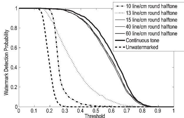
Figure 7 Watermark detection probabilities for the different frequencies of a round halftone Slika 7. Vjerojatnost detekcije vodenog znaka za različite linijature točkastog rastera
