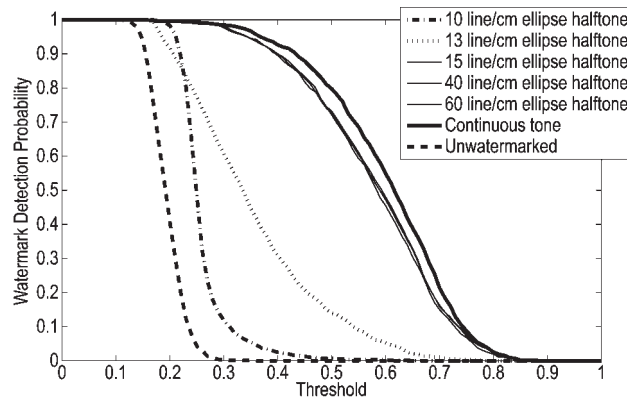
Figure 8 Watermark detection probabilities for the different frequencies of an ellipse halftone Slika 8. Vjerojatnost detekcije vodenog znaka za različite linijature eliptičnog rastera
