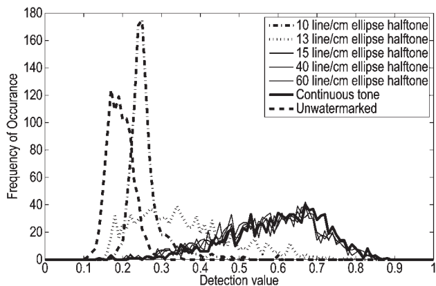
Figure 11 Histogram of detection values for an ellipse halftone Slika 11. Histogram detektiranih vrijednosti za eliptični raster
