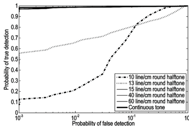
Figure 13 ROC curve for a round halftone Slika 13. ROC krivulja za točkasti raster
