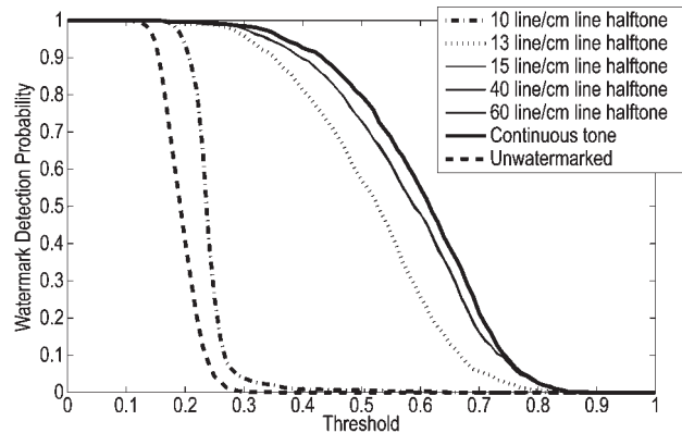
Figure 9 Watermark detection probabilities for the different frequencies of a line halftone Slika 9. Vjerojatnost detekcije vodenog znaka za različite linijature linijskog rastera
