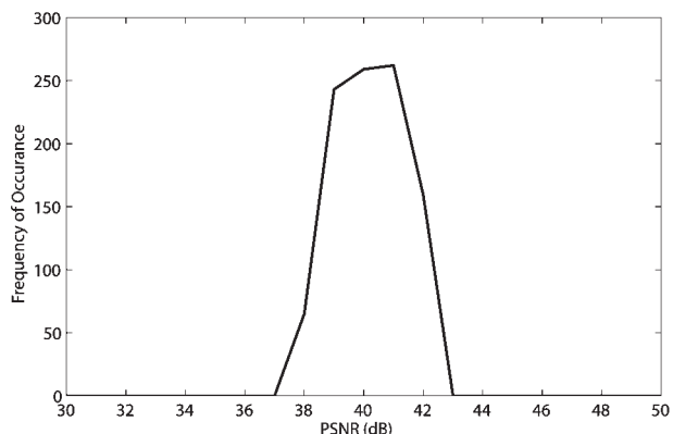
Figure 5 Histogram of the PSNR values of watermarked images Slika 5. Histogram PSNR vrijednosti označenih slika
