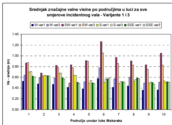
Slika 13. Srednjak značajne valne visine po područjima u luci - VARIJANTA 1. i 3.
