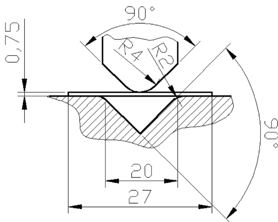
Figure 1. V-die tool for sheet metal bending Slika 1. V-alat za savijanje lima
