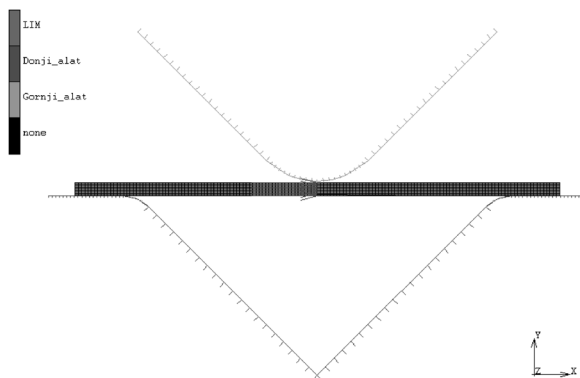
Figure 4. FEM model of 90° V-die bending tool from Figure 1 Slika 4. MKE model alata za savijanje s kutom od 90° koji je prikazan na Slici 1
