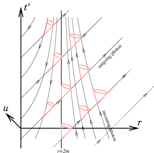
Figura 3: Spazio-tempo di Schwarzschild in coordinate di Eddington-Finkelstein ritardate
