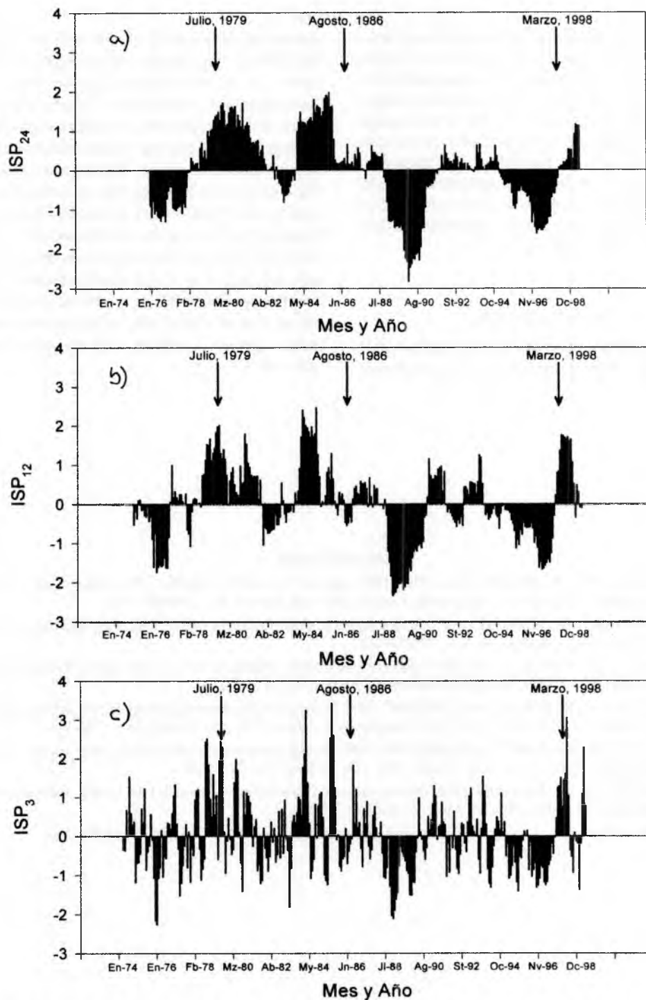
Figura 2. Valores de ISP para Río Cuarto calculados de la serie 1974/99 para periodos de a) 24 meses ( ISP_{24} ); b) 12 meses ( ISP_{12} ); c) 3 meses ( ISP_3 ) y fechas de ocurrencia de inundaciones a lo largo de la serie (flechas)
