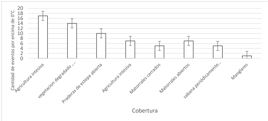
Figura 9. Cantidad de eventos con T_s superior a 0 de acuerdo a la cobertura del suelo
