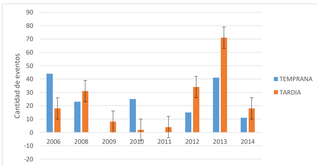
Figura 15. Conteo de eventos de heladas tempranas y tardías por año.
