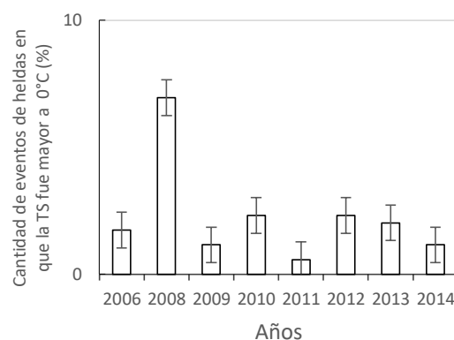
Figura 7. Porcentaje anual de datos de temperatura Ts por encima de 0°C para heladas detectadas mediante Ta.
