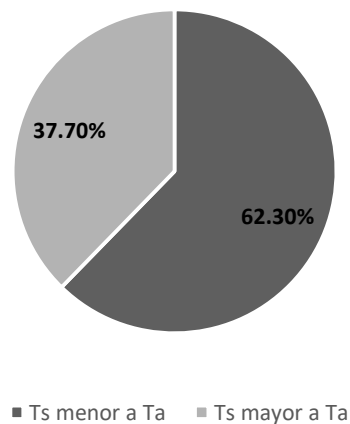
Figura 10. Porcentaje de datos de temperatura T_s mayor a T_a para todo el periodo de estudio 2006-2014.
