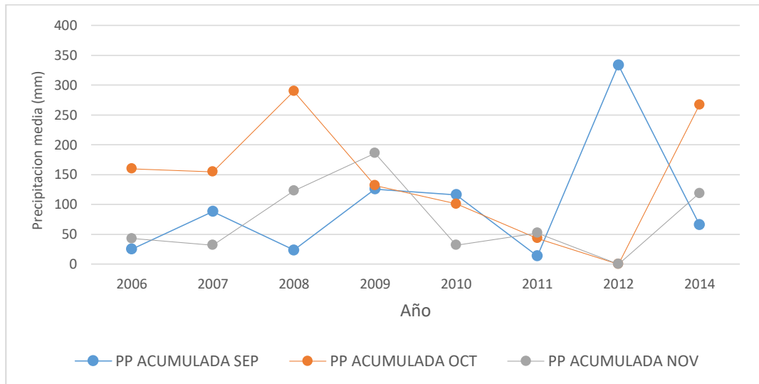
Figura 13. Gráfico comparativo del 2006 al 2014 entre los valores promedio de precipitación acumulada para septiembre, octubre y noviembre.
