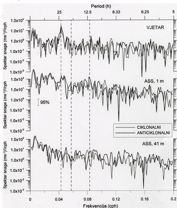
Slika 6. Rotacijski spektri (ciklonalni i anticiklonalni) vjetra u Opatiji i morskih struja na postaji ASS-1 na dubinama 1 m i 41 m u Podurinj, srpanj 1999. godine.
