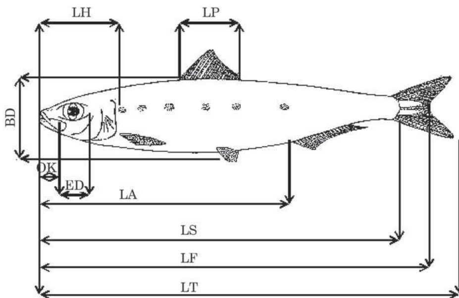
Figure 2. Analyzed morfometric parametres of sardine Slika 2. Analizirana morfometrijska obilježja srdele
