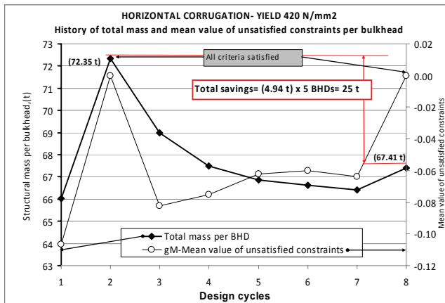
Figure 16 HC variant – History of structural mass with the mean value (gM) of unsatisfied constraints for the final optimization run Slika 16 HC varijanta – Promjena strukturne mase te srednje vrijednosti (gM) kroz projektne cikluse za finalnu optimizaciju
