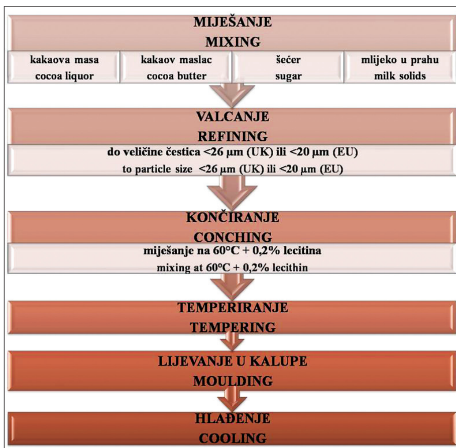
Slika 2. Klasičan shematski prikaz proizvodnje čokolade (Kelly, 2006)
