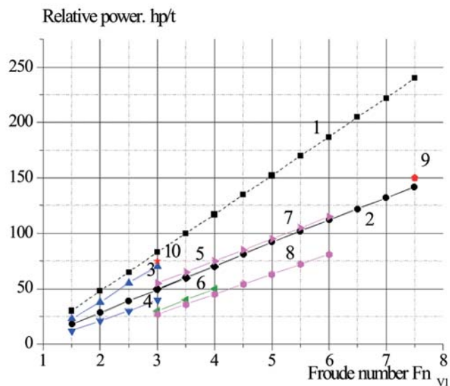
Slika 2 Relativna snaga (po toni pune istisnine): 1,2 – jednotrupci, gornja i donja granična vrijednost; 3,4 – katamarani; 5,6 – barke s krilcima; 7,8 – barke na zračnom jastuku, 9 – trimaran „sječač valova“ razvijen iz istovrsnog katamarana; 10 – „poluglisirajuća“ SWA barka
