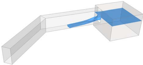
Slika 4. Vodno lice u 3D modelu u trenutku t=1 s
