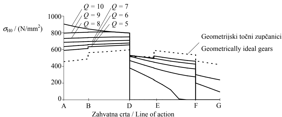
Slika 6. Raspodjele napreznja na boku zuba zupčanika Figure 6. Contact stress distributions in gears
