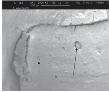
Slika 2. Reprezentativna slika konvencionalnog stakleno-ionomernog cementa Fuji IX nakon 18 mjeseci u umjetnoj slini – SEM (sekundarni elektronički način)- praznine su ispunjene sferičnim tijelima Figure 2 Representative image of a conventional glass-ionomer cement Fuji IX after 18 month storage in artificial saliva – SEM (secondary electron mode): air voids filled with spherical bodies
