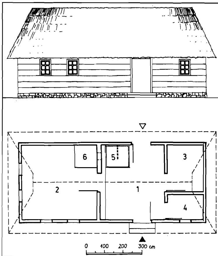
SL. 10. TRADICIONALNA KUĆA U SELU HRSINI: A - GLAVNI ULAZ; B - GOSPODARSKI ULAZ; 1 - KUHINJA UGLJENICA; 2 - HIŽA; 3 - HIŽICA; 4 - SPREMIŠTE; 5 - OGNJIŠTE; 6 - VELIKA PEĆ
