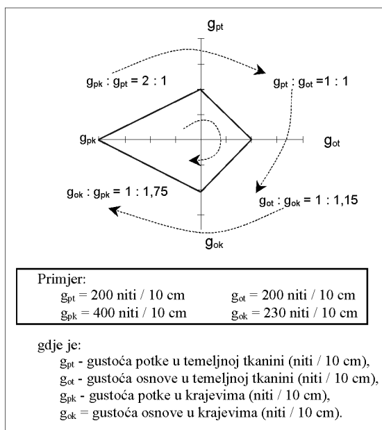
Sl.8 Odnos gustoća temeljne tkanine i krajeva kada je g_{pt} \cdot g_{ot} = 1:1
