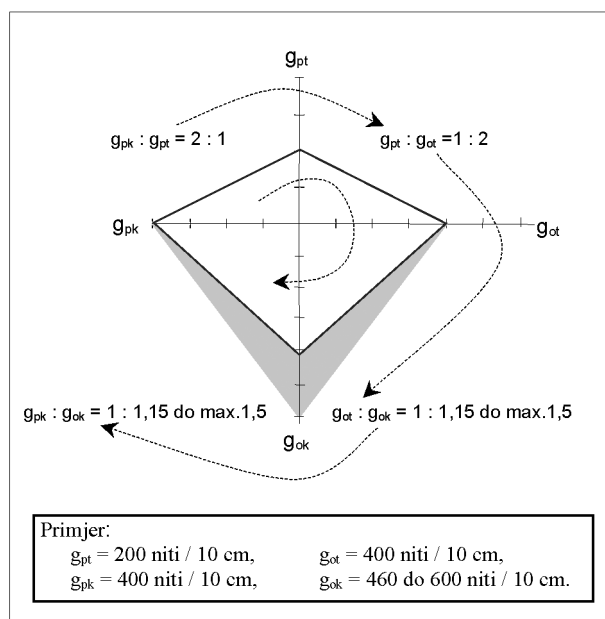
Sl.9 Odnos gustoća temeljne tkanine i krajeva kada je g_{pt} \cdot g_{ot} = 1:2
