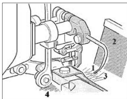
Sl.2 Uređaj za tvorbu uvučenih krajeva: 1 - igla za uvlačenje niti u krajeve, 2 - brdo, 3 - zijev, 4 - tkanina
