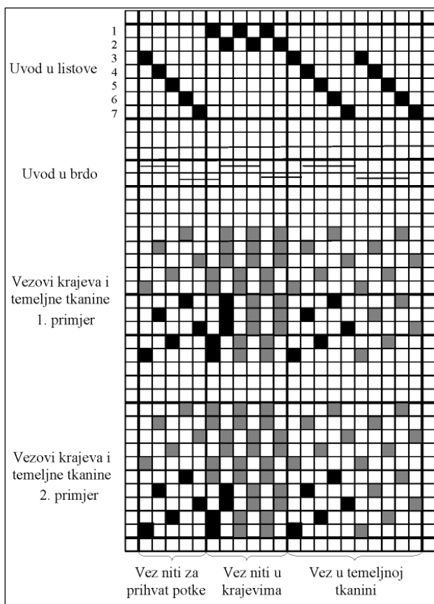
Sl.7 Uzornica krajeva i temeljne tkanine 5-vezni potkin atlas A 1/4 D (2)
