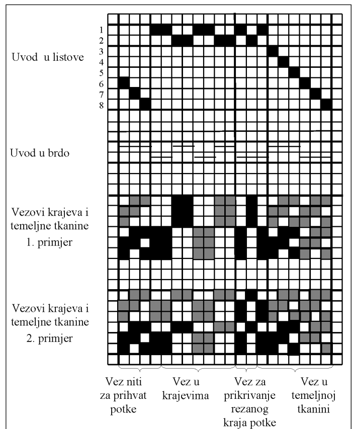
Sl.5 Uzornica krajeva i temeljne tkanine za keper K 2/1 D
