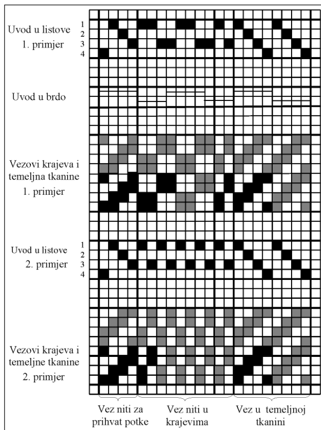
Sl.6 Uzornica krajeva i temeljne tkanine za keper K 2/2 D (cirkas)
