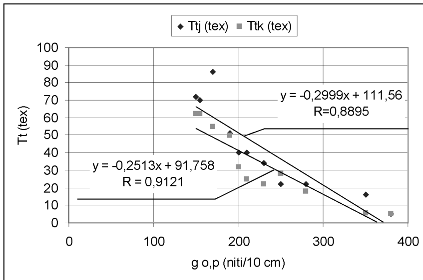
Sl. 10 Odnos finoće i gustoće pređe u tkanini (prema sl.8) s prikazanim pravcima regresije i koeficijentima korelacije (R); Ttk – finoća končane pređe (tex), Ttj – finoća jednonitne pređe (tex), R – koeficijent korelacije
