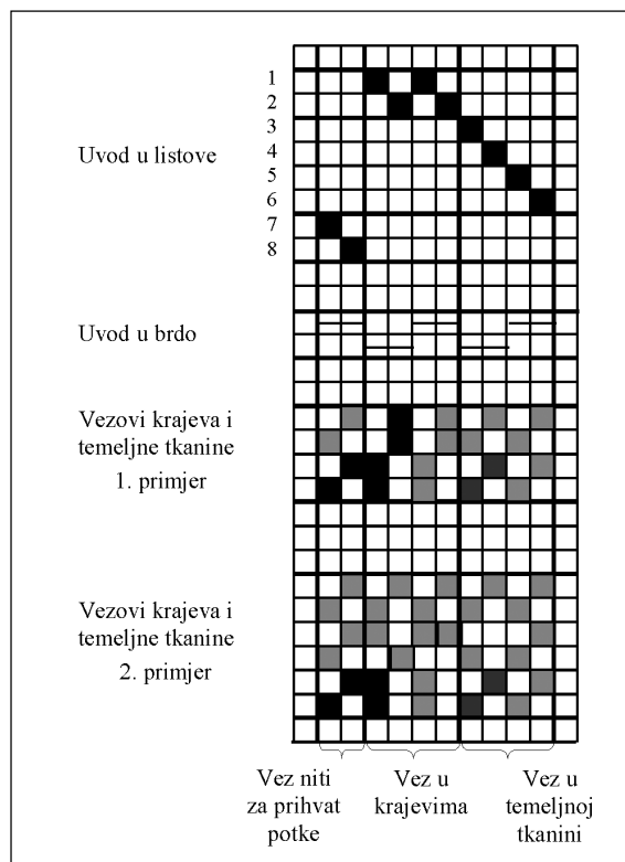
Sl.4 Uzornica krajeva i temeljne tkanine za platno
