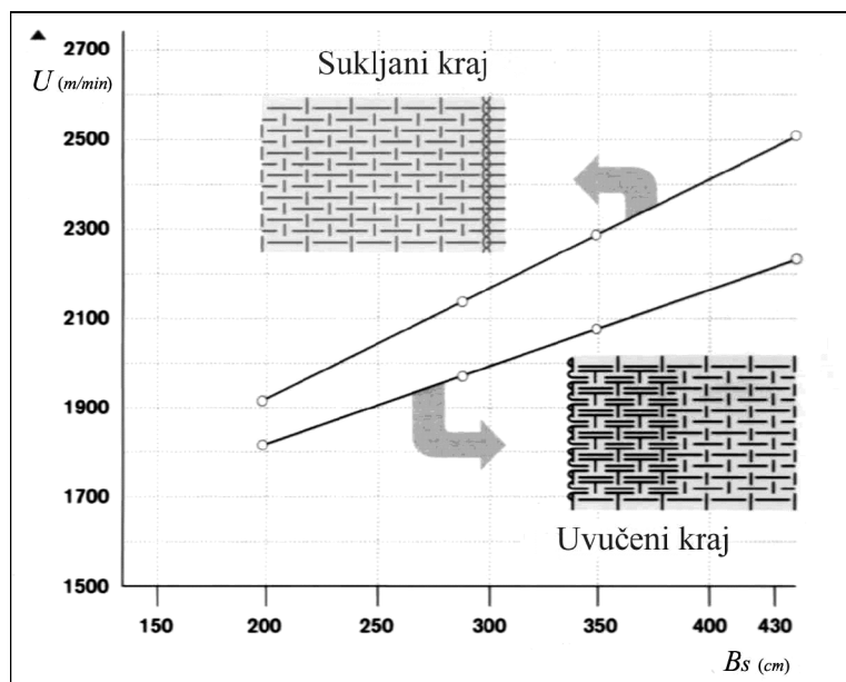
Sl.1 Ovisnost utkivnog učinka o radnoj širini stroja za različite oblike krajeva: U - utkivni učinak stroja, B_s - radna širina stroja [3]
