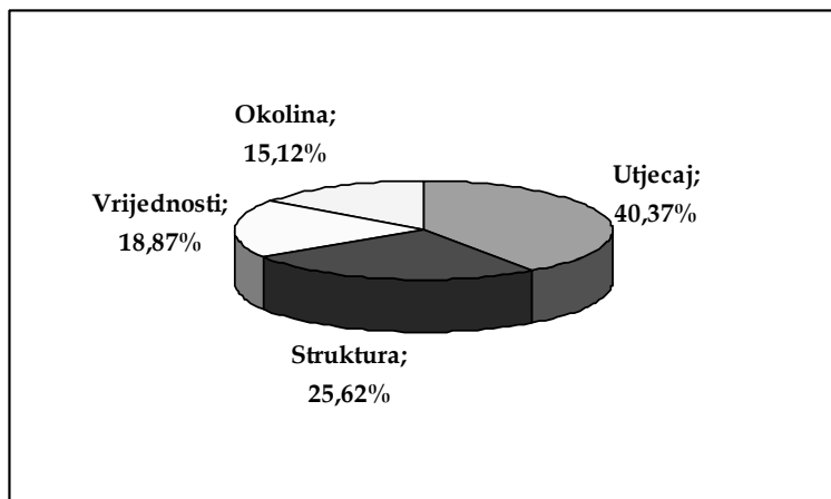
Grafikon 1: Distribucija indikatora ukupnoga uzorka po dimenzijama
