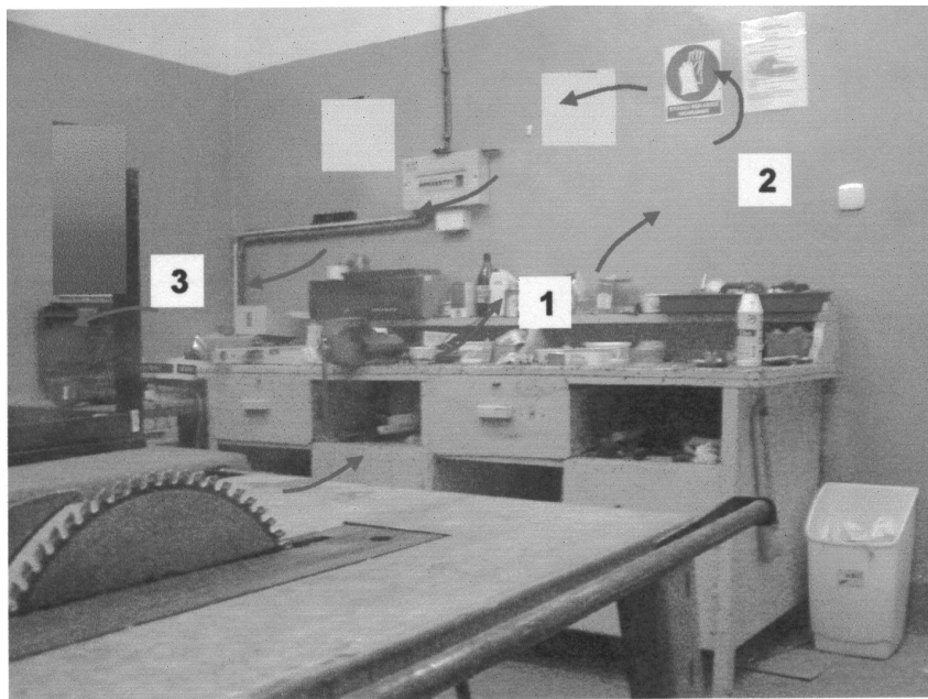
Figure 2. Visualisation of smoke flow in the pollution dispersion area in the working room Slika 2. Vizualizacija gibanja dima u području širenja zagađenja u radnoj prostoriji
