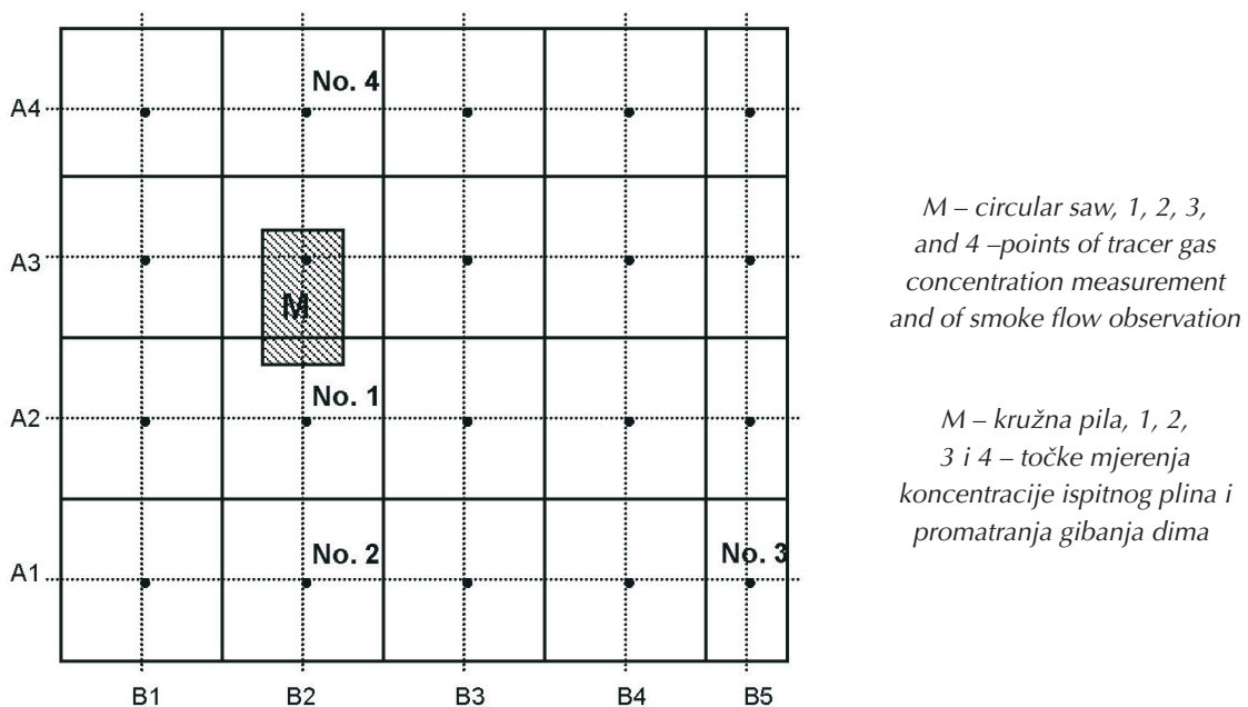
Figure 3. Measurement points distribution in the working room Slika 3. Razmještaj mjernih točaka u radnoj prostoriji
