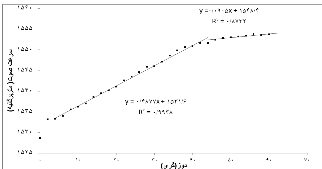
شکل ۳. حساسیت در بازه 44-60 گری برای پارامتر سرعت انتشار صوت بر حسب متر بر ثانیه
