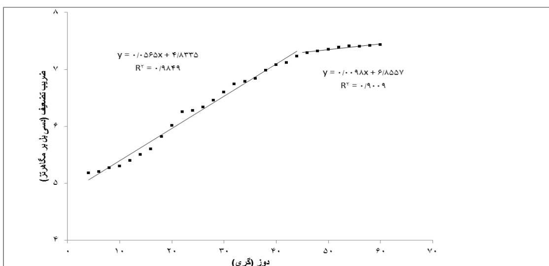
شکل ۴. حساسیت در بازه 44-60 گری برای پارامتر ضریب تضعیف صوت بر حسب دسی بل بر مگاهرترز
