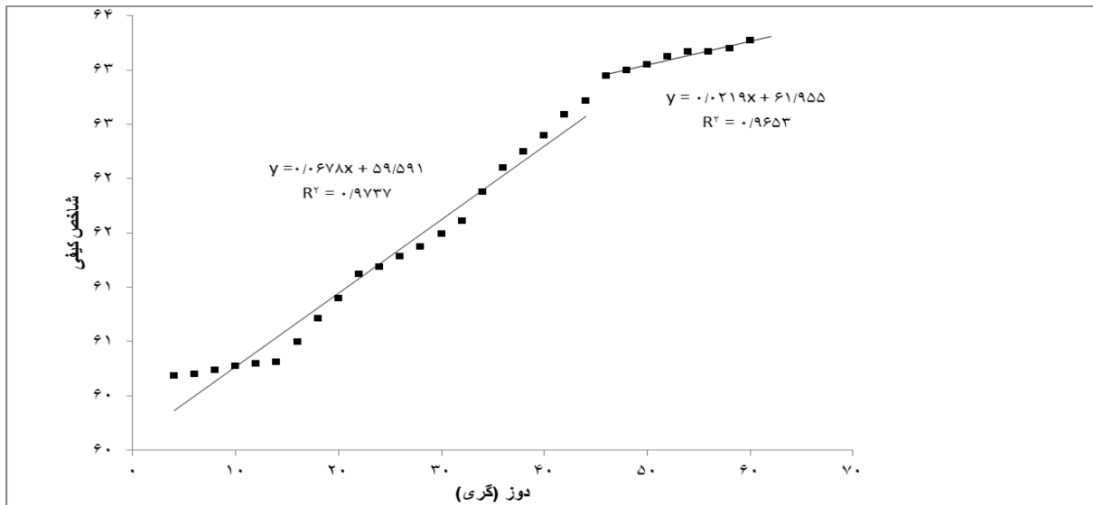
شکل ۵. حساسیت در بازه ۱۰-۴۸ گری برای پارامتر شاخص کیفی
