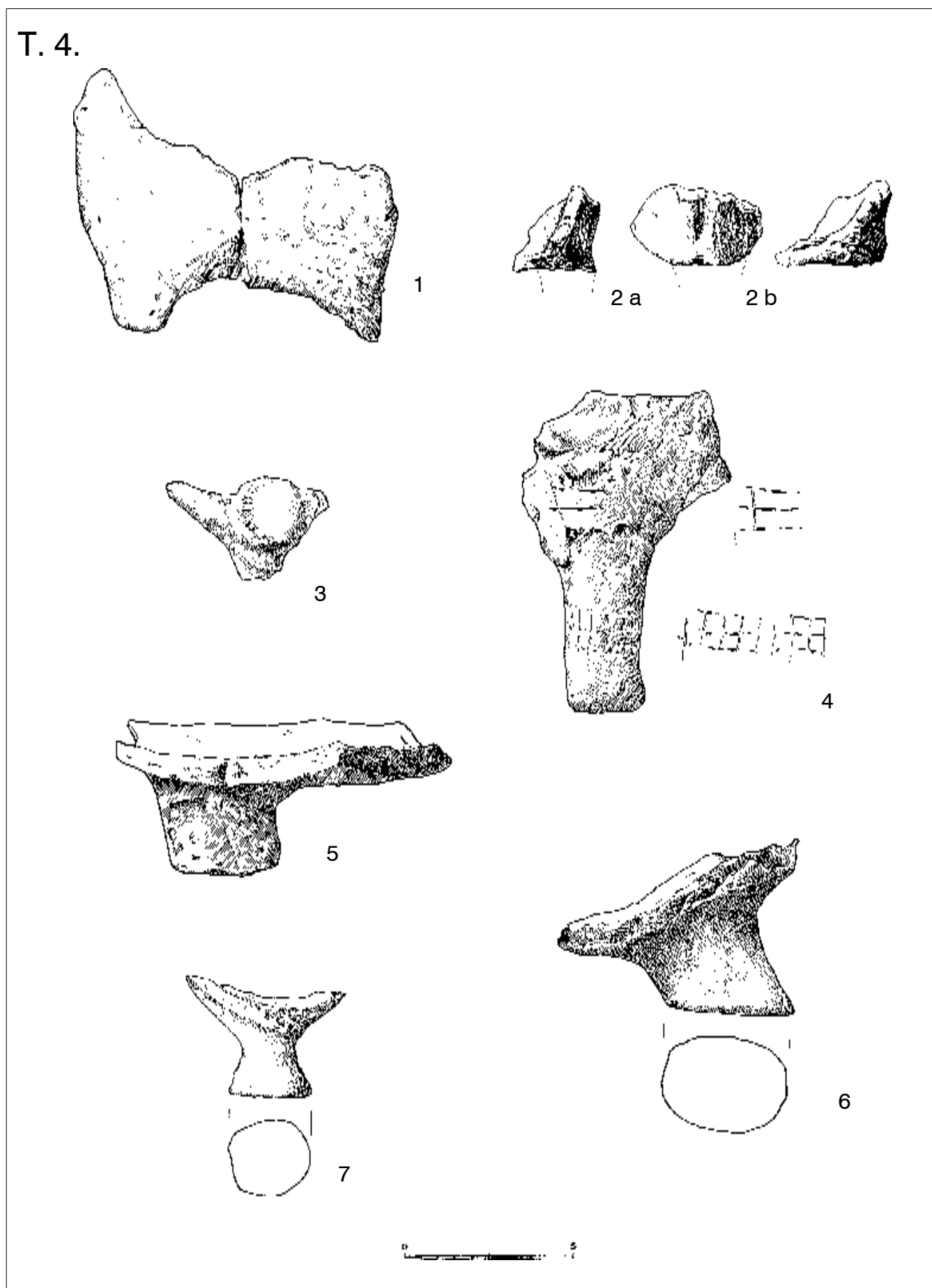
T. 4. Slavonski Brod - Galovo, žrtvenici tipa 4, 5, 6 (crtež M. Gregl)
