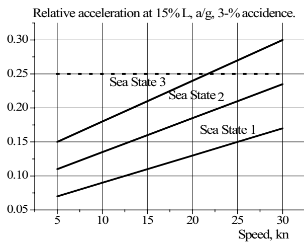
Figure 12 Relative vertical acceleration a/g at 15%L from FP, 3% accidentence Slika 12 Relativno vertikalno ubrzanje a/g na 15%L od prednje okomice, 3% premašaja
