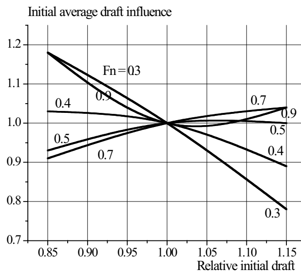
Slika 4 Primjer utjecaja početnoga srednjeg gaza na koeficijente preostalog otpora tradicionalnog SWATH-a (konstantna istisnina)
