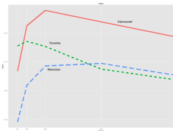
C:0.30,D:0.00,UH:0.70
