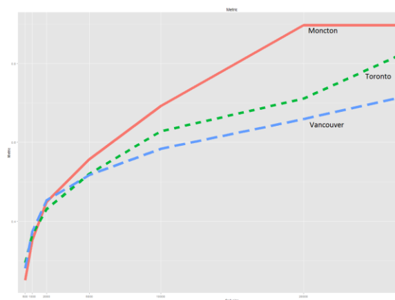
C:0.8,D:0.10,UH:0.10
