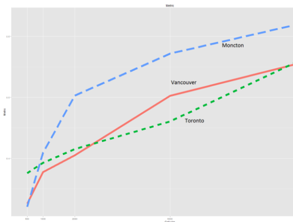
C:0.33,D:0.33,UH:0.33
