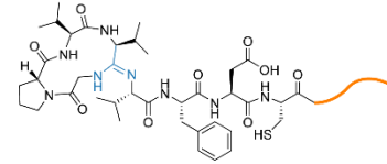
macrolactamidine
