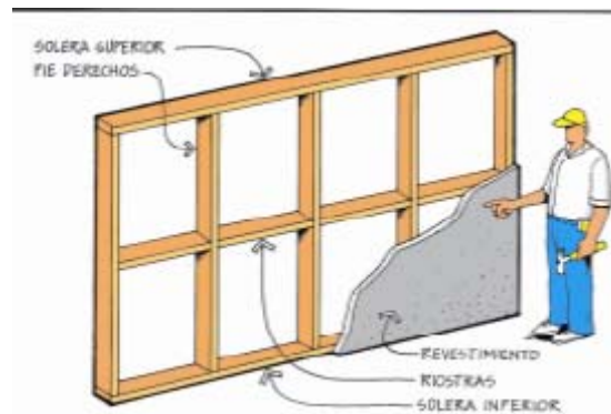
Figura 2. Nomenclatura sistema estructural Bahareque encementado (AIS, 2000).
