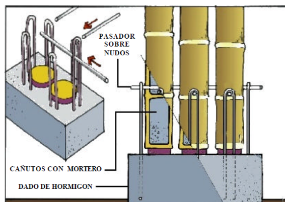
Figura 5. Conexiones para columnas de más de una guadua (NSR-10, apéndice E-B.3)
