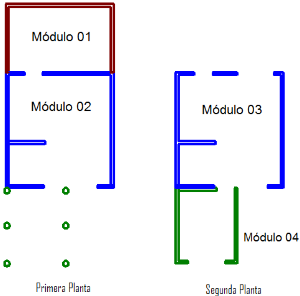
Figura 3. Configuración estructural del diseño en bahareque encementado
