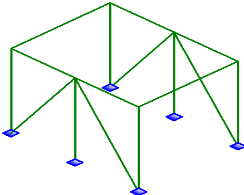
Figura 4. Configuración estructural de soporte módulo 04, pórtico en guadua.
